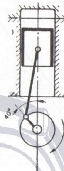
Fig. 33 - Schema dell'anticipo all'accensione.
