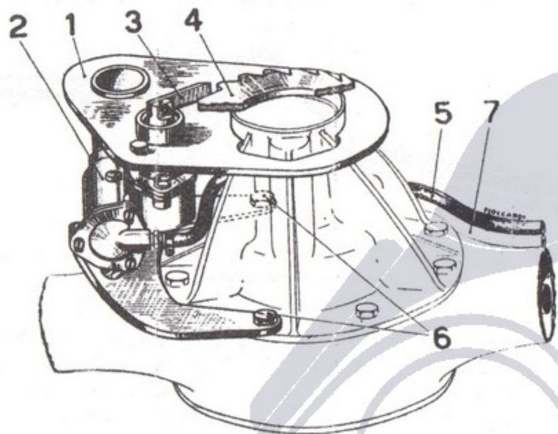
Fig. 97 - Il « Retrobloc Modauto » applicato alla trasmissione della « 500 ».
