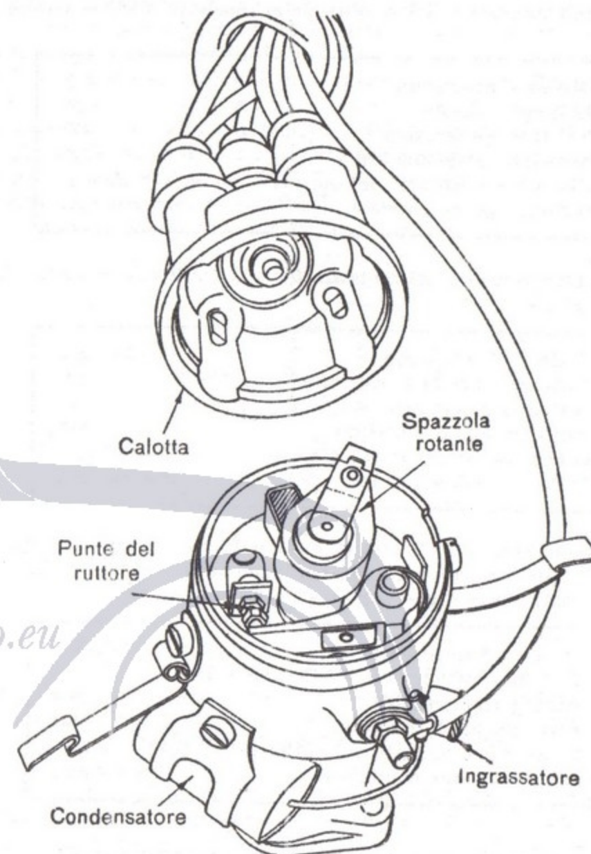
Fig. 32 - Interno del distributore d'accensione Magneti Marelli della «500». Un'apposita tacca obbliga a rimontare la calotta in modo esatto. Sulla calotta sono indicati con numeri i cilindri ai quali ciascun cavo deve essere collegato. Dal motore n. 330801 il distributore è provvisto di correttore d'anticipo a depressione.
