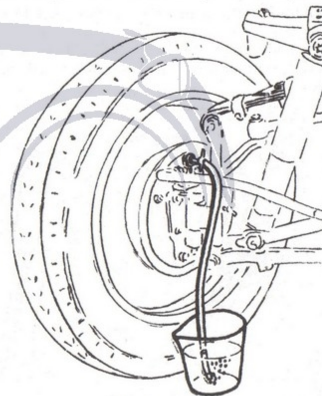
Fig. 52 - Spurgo dell'aria dalle tubazioni del comando idraulico dei freni. Per questa operazione sono necessari uno speciale raccordo, un tubetto di gomma lungo 30 cm circa ed un bicchiere trasparente e pulito. Il liquido che esce dal tubetto non deve essere riutilizzato.
