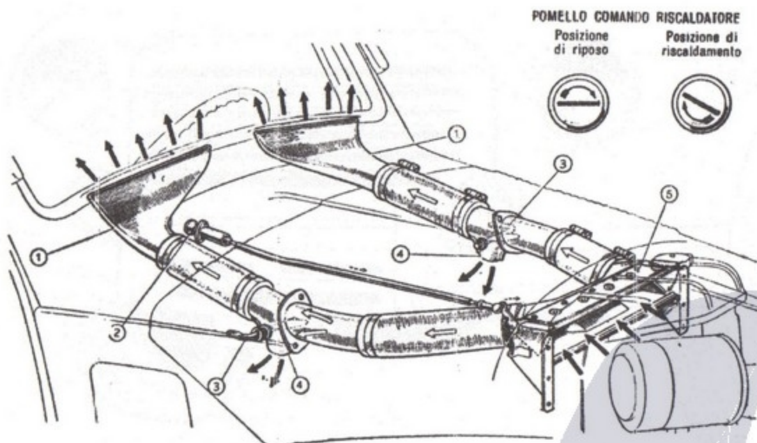
Fig 75 - L'impianto di riscaldamento e sbrinamento della «500» C.
