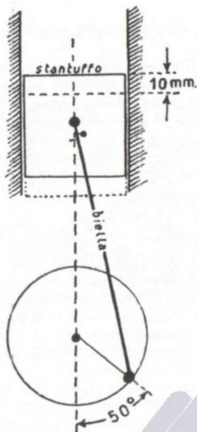
Fig. 89 - Per controllare se la distribuzione del motore FIAT «500» a valvole laterali è in fase (motore montato sulla vettura) ci si serve del cilindro n. 4, riscontrando se 50° prima del P.M.I. la valvola di scarico (regolata provvisoriamente con gioco di 0,25 mm.) comincia ad aprirsi.
