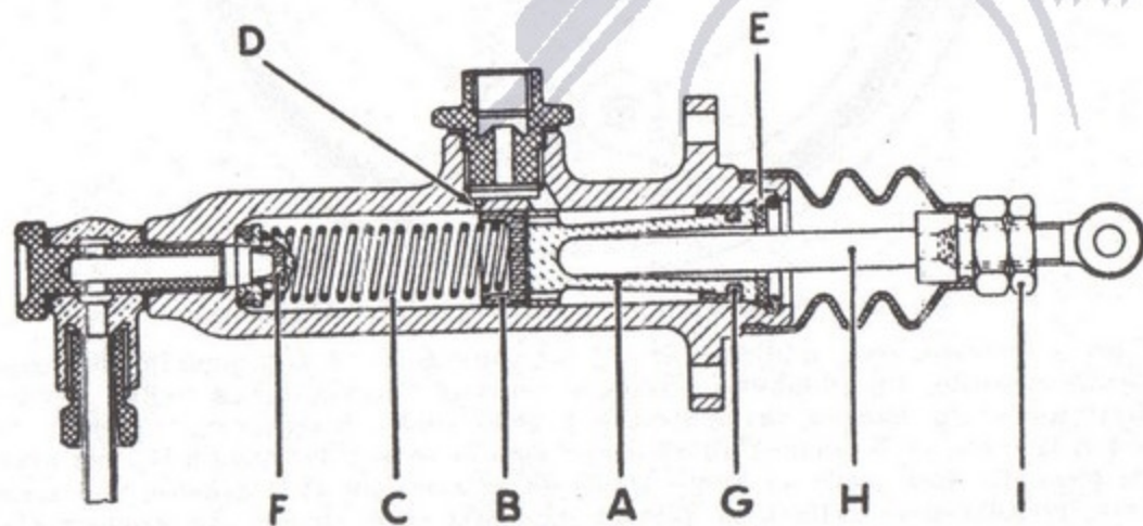
Fig. 49 - Sezione della pompa del comando idraulico dei freni tipo « Lockheed ». A, Stantuffo; B, Calotta di tenuta; C, Molla di richiamo; D, Foro di compensazione del liquido; E, Arresto della posizione di riposo; F, Valvola; G, Seconda calotta di tenuta; H, Stelo di comando; I, Dadi per la regolazione della corsa.
