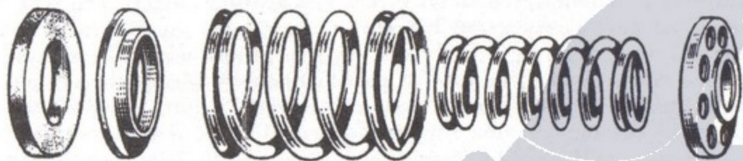
Fig. 65 - Le molle speciali per valvole ABARTH sono dotate di appositi scodellini alleggeriti e di rosette di materiale antivibrante.
