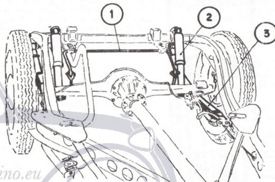
Fig. 43 - La sospensione posteriore della « 500 » B e C.
