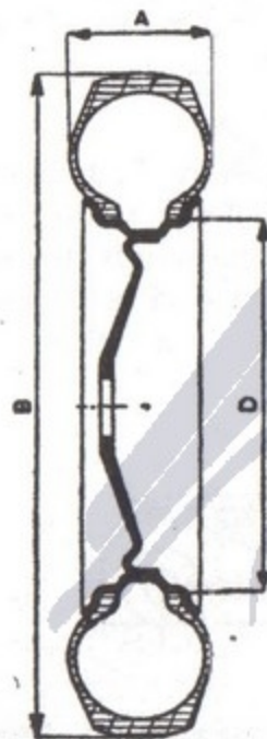
Fig. 2 - Sezione di una ruota gommata per autovettura.
