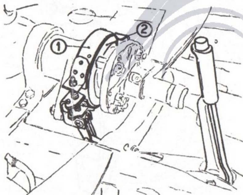
Fig. 53 - Freno sulla trasmissione comandato da leva a mano.
