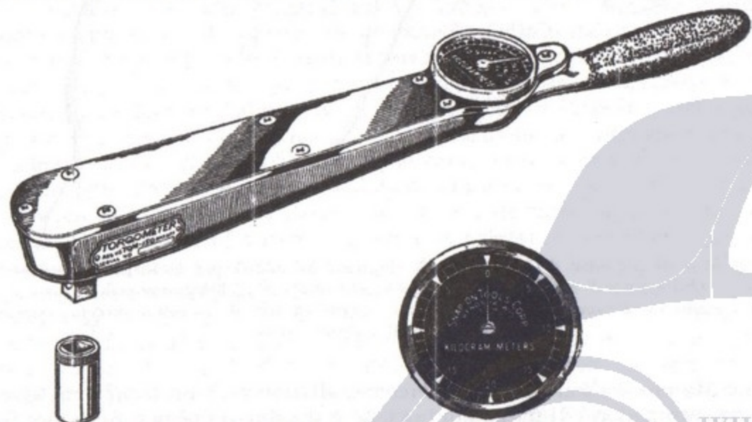
Fig. 82 - La misurazione esatta del momento torcente applicato ad un bullone può ottenersi solamente con l'impiego di una « chiave dinamometrica »: in figura, la SNAP-ON TORQUEMETER americana.
