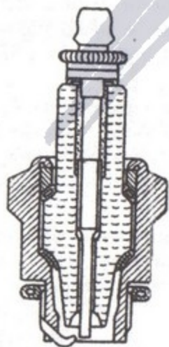
Fig. 6 - Sezione di una candela d'accensione.
