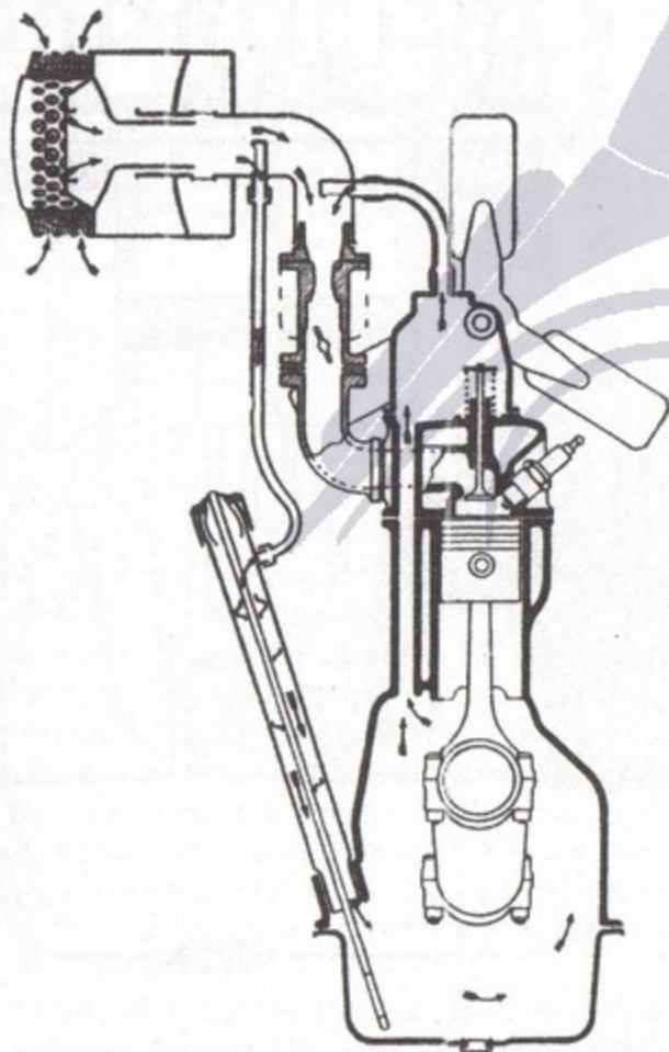
Fig. 15 - Schema dell'impianto di ventilazione interna del motore.
