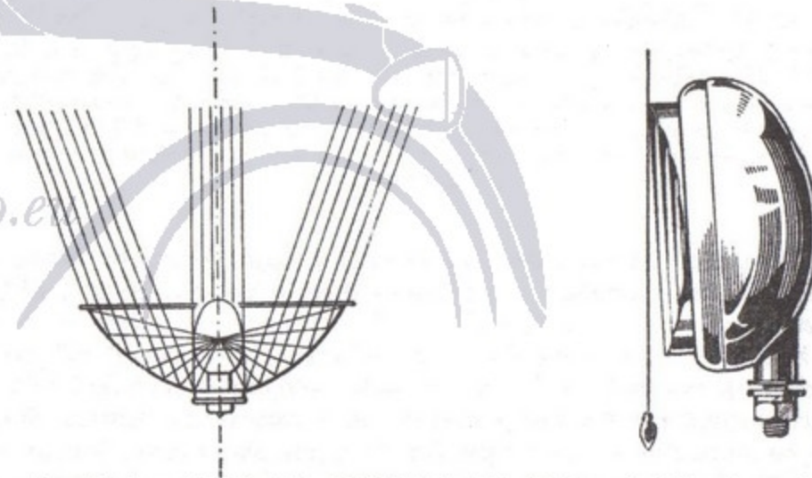
Fig. 74 - Il proiettore fendinebbia CARELLO P.F. 51 ben s'adatta al montaggio in coppia sulla « 500 ».
