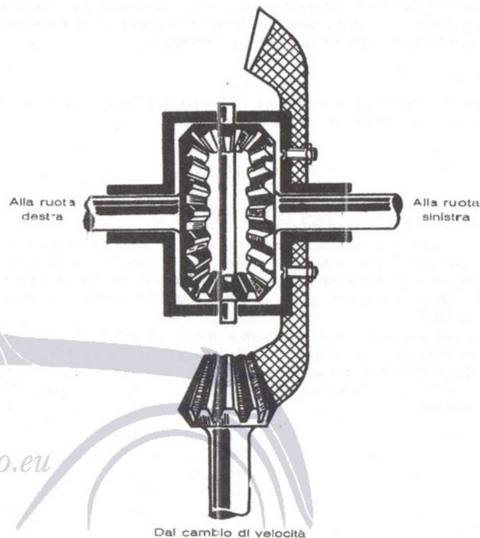
Fig. 8 - Gruppo conico e differenziale.
