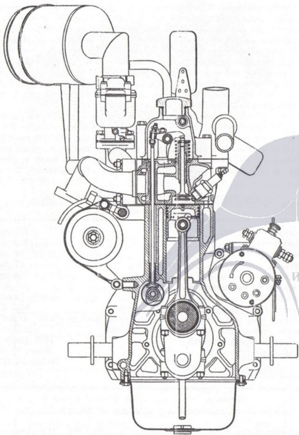
Fig. 12 - Sezione trasversale del motore della vettura FIAT «500» B. La testata è di ghisa.
