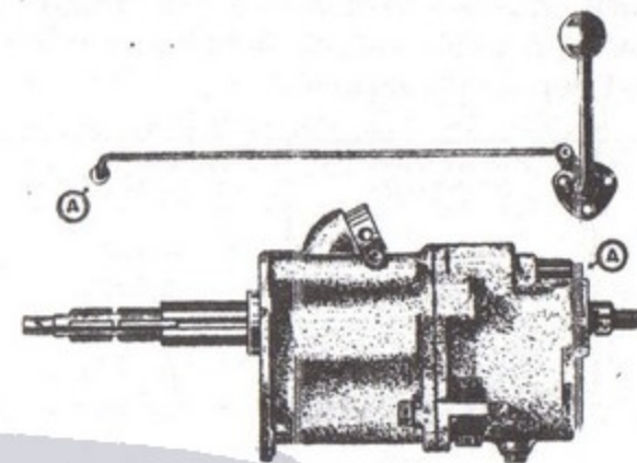
Fig. 68 - Moltiplicatore di velocità MONVISO (rapporto 1/1,26) per Fiat «500».
