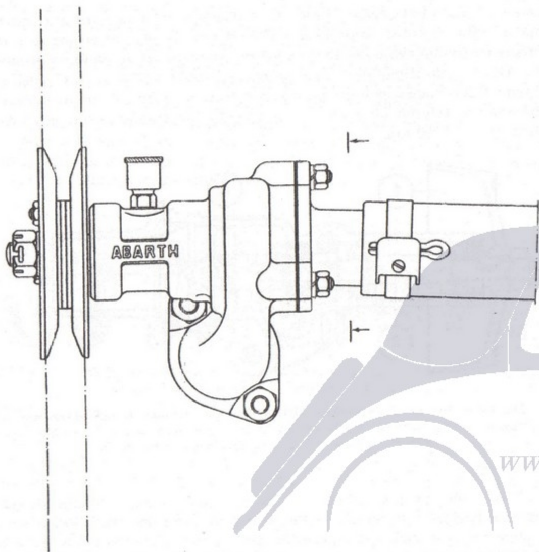
Fig. 67 - Pompa acqua speciale ABARTH tipo 51 per motori delle vetture Fiat «500» A, B e C.
