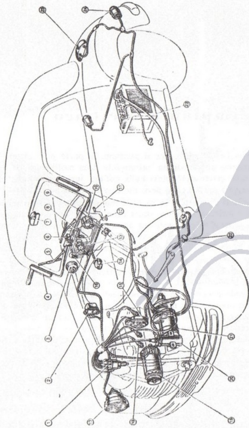
Fig. 28 - L'impianto elettrico della FIAT «500» C.
