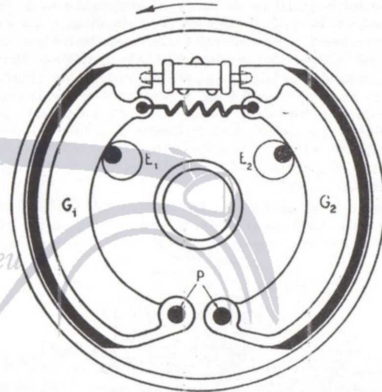
Fig. 48 - Freno a tamburo comandato idraulicamente.
