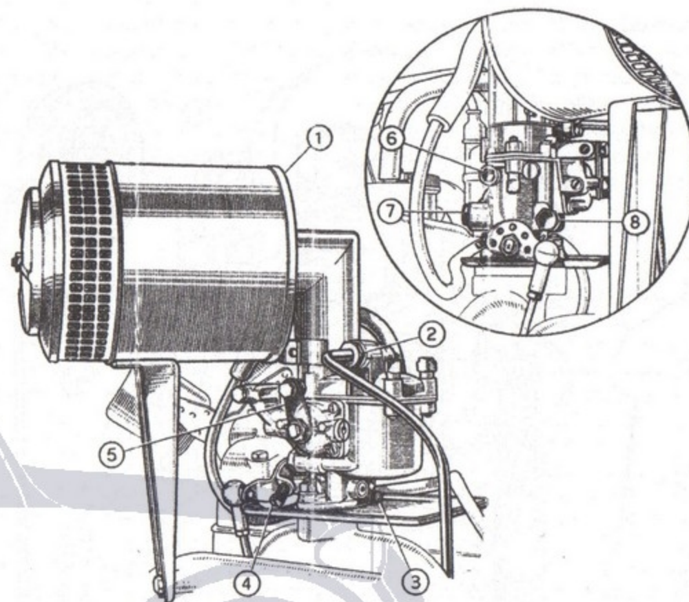
Fig. 19 - Carburatore «Solex» 22 IAC.
