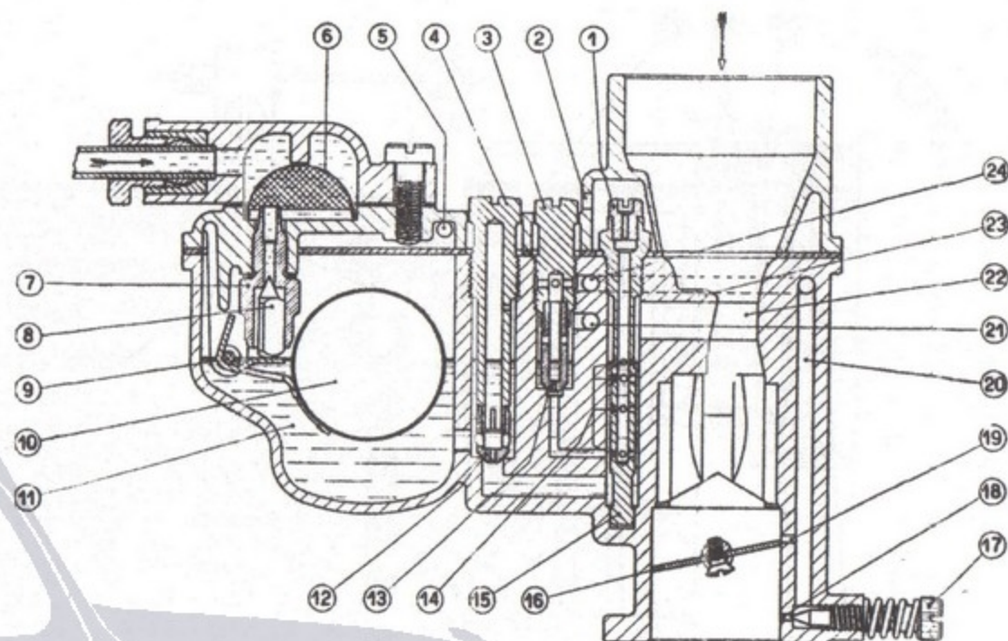
Fig. 17 - Carburatore «Weber» 22 DRS.
