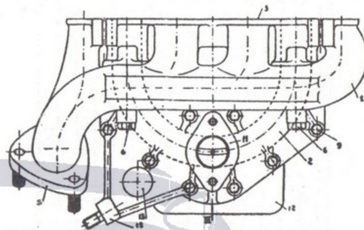
Fig. 94 - Sezione del collettore monocarburetor « Modauto » per FIAT « 500 » B e C. Il condotto semicircolare è quello d'aspirazione, mentre quello rettilineo è il collettore di scarico.
