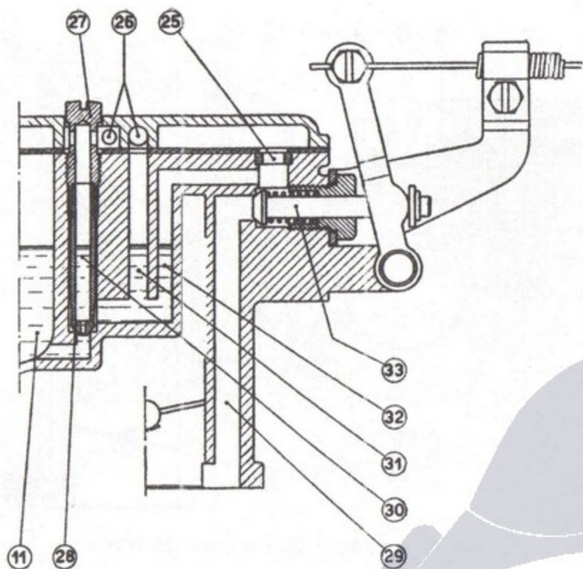
Fig. 18 - Dispositivo d'avviamento del carburatore «Weber» 22 DRS.
