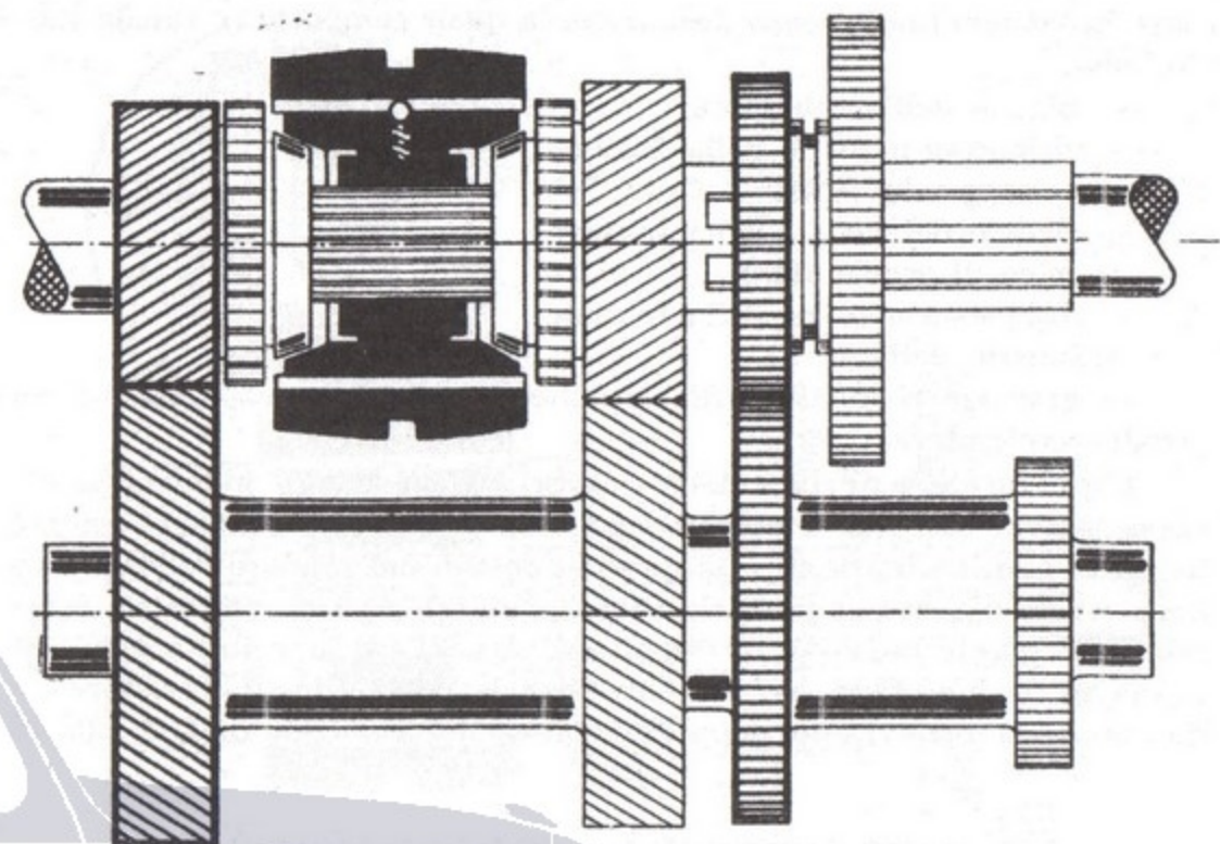
Fig. 24 - Il cambio in posizione di 2ª velocità - Il moto passa dall'albero primario a quello ausiliario per mezzo della coppia di ingranaggi sempre in presa (ingranaggi silenziosi), il passaggio dall'ausiliario al secondario avviene attraverso la coppia della seconda velocità (ingranaggi a denti diritti).
