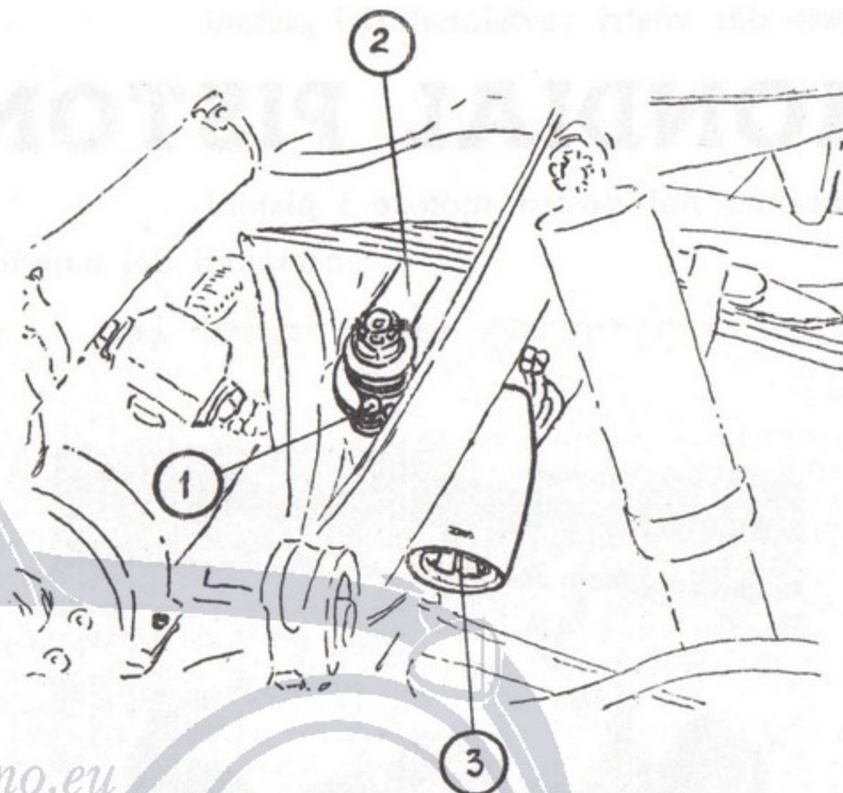
Fig. 57 - Regolazione del gioco del meccanismo di guida.
