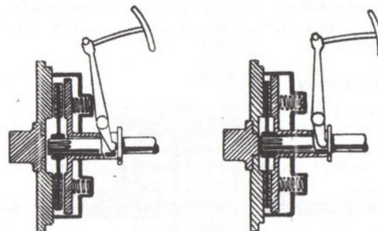
Fig. 7 - Sezione di una frizione monodisco a secco.
