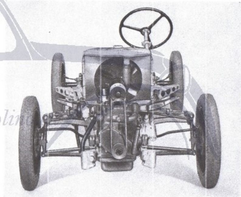
Fig. 7. - Autotelsio mod. 500 visto anteriormente.
