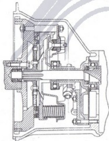
Fig. 54. - A - Attrezzo A. 10112 per smontaggio, rimontaggio e registrazione della frizione. S - Anelli di spessore.
