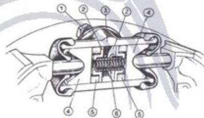
Cilindro comando idraulico freni « Brevetto FB ».
