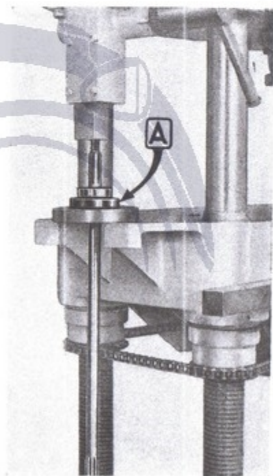
Fig. 74. Smontaggio alberi differenziale con estrattore A. 6466.
