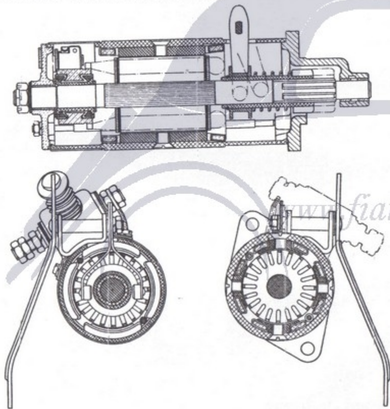
Fig. 134. - Sezioni del motorino d'avviamento (montato fino al N. 033508 di motore).
