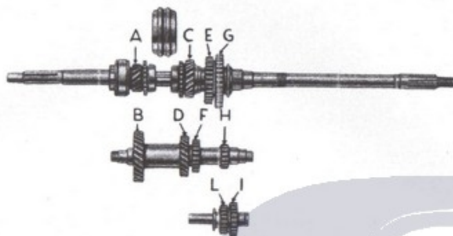
Fig. 67. - Disposizione degli alberi ed ingranaggi del cambio.
