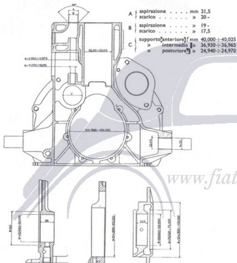
Fig. 21. - Dati principali del gruppo cilindri.
