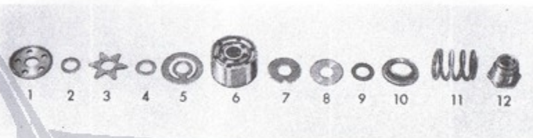
Fig. 175. - Particolari della valvola di rimbalzo di un ammortizzatore. I numeri corrispondono all'ordine nel quale devono essere infilati nello stelo dell'ammortizzatore.
