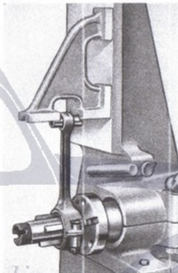
Fig. 33. - Controllo allineamento bielle sull'apparecchio C. 627.
