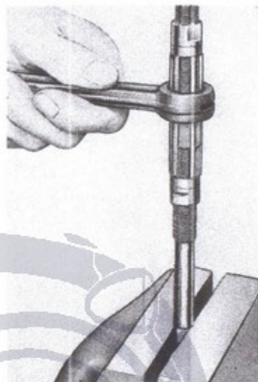
Fig. 34. - Ripassatura della boccola nel piede di biella mediante il liscioio a lame regolabili U. 0326.
