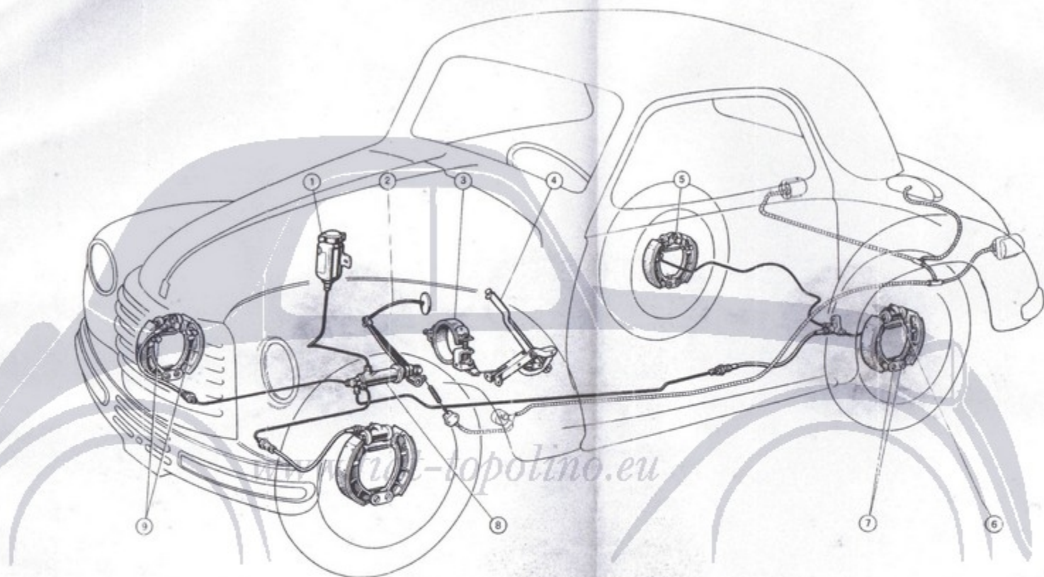
Fig. 189. - Schema dei freni idraulici alle ruote e meccanico sulla trasmissione.
