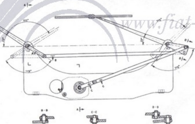
Fig. 191. - Disposizione del meccanismo per il comando delle racchette tergicristallo.
