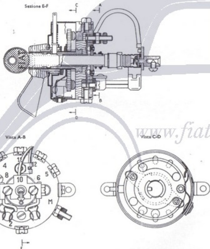
Fig. 139. - Schema, sezione e viste del quadretto (montato fino alla vettura N. 019839).
