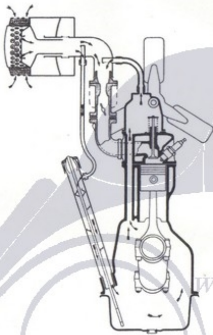
Fig. 159. - Schema della ventilazione interna del motore.
