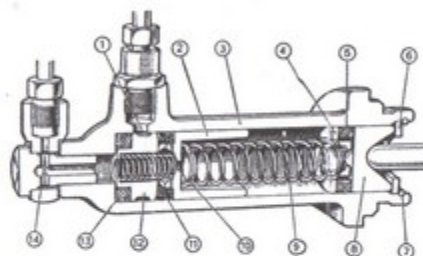
Fig. 106. Pompa di comando idraulico freni « Brevetto FB ».
