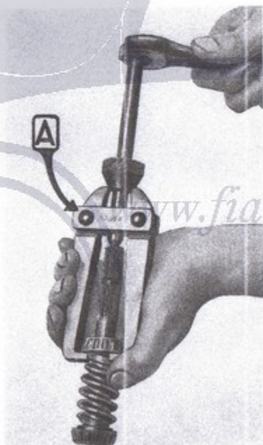
Fig. 97. - A = Estrattore A. 6514 per anelli interni cuscinetti a rulli sulla vite perpetua comando guida.
