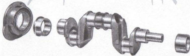
Fig. 25. - Albero manovella e cuscinetti di banco.
