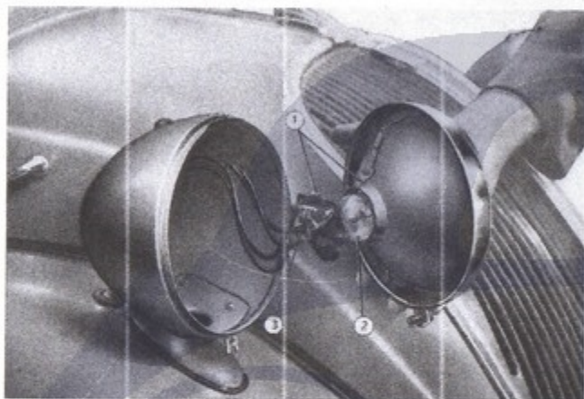
Fig. 184. - Smontaggio del supporto delle lampadine dai proiettori.
