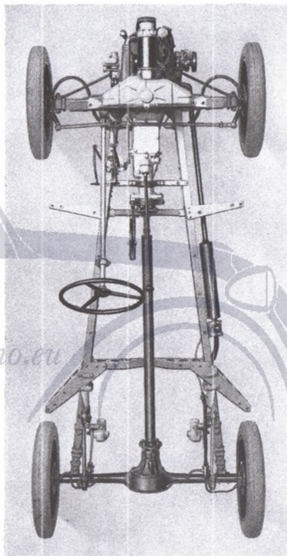
Fig. 3. - Autotelaio mod. 500 fino al N. 046000, visto dall'alto.
