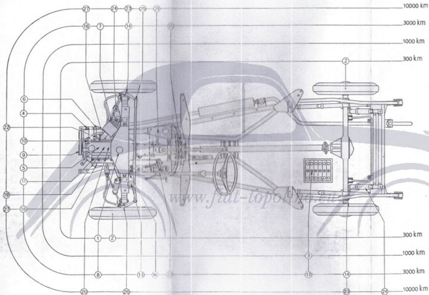
Fig. 186. - Schema delle pulizie, verifiche
