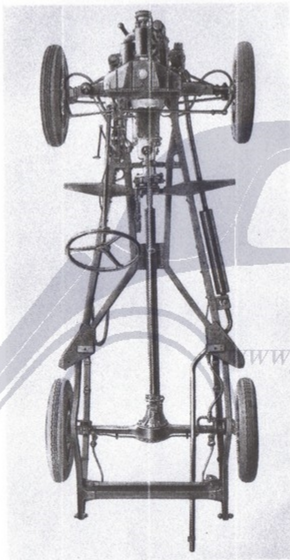
Fig. 4. - Autotelaio mod. 500 dal N. 046001, visto dall'alto.
