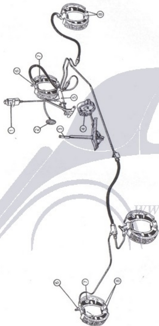
Fig. 105. - Schema dei freni.
